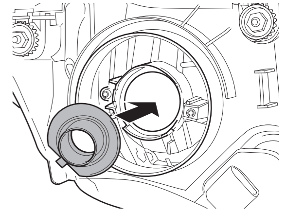
図4. フランジ組付要領
