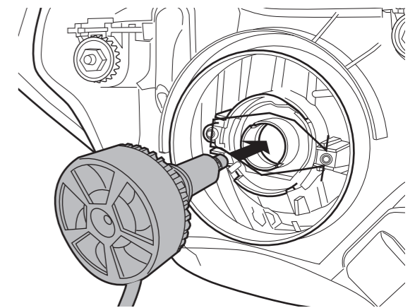
図5. LEDバルブ取付要領
