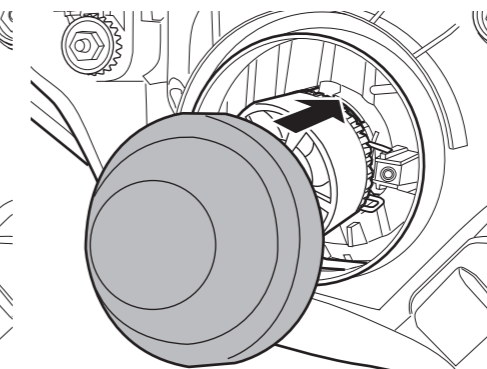
図7. ゴムカバー取付要領
