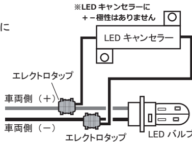
LED キャンセラー接続図 (並列接続)
